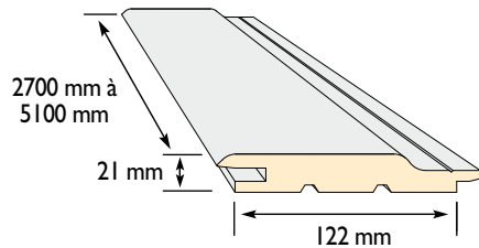
Profil Façade (Epicéa)
