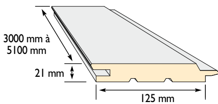
Profil Néliö (Epicéa)
