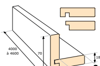
Profil d'angle réversible AB non resséché : 70 x 18 selon longueur disponible
